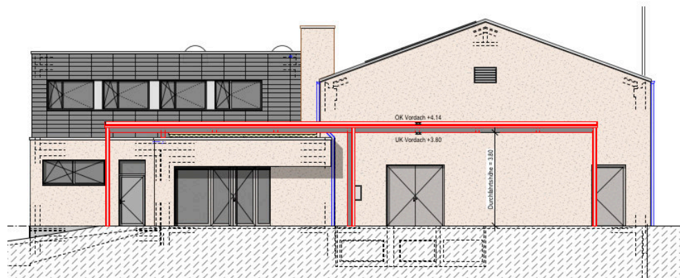
ANSICHT
